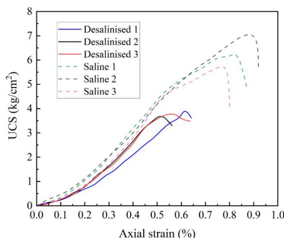
شکل ۹. تأثیر میزان نمک بر رفتار تنش-کرنش نمونه‌های بهسازی شده فاقد نمک و نمونه‌های دارای نمک
