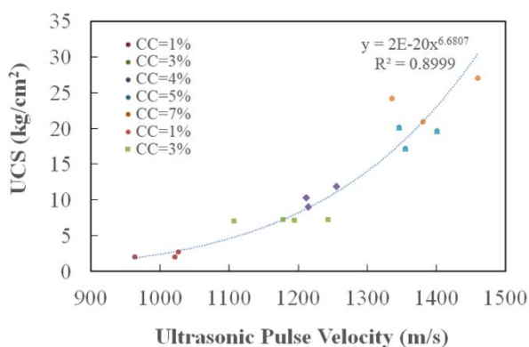
شکل ۴. ارتباط بین مقاومت تک محوری با سرعت موج اولتراسونیک در نمونه‌های با دانسیته نسبی ۷۰٪ و درصد سیمان‌تاسیون ۱ تا ۷٪ Fig. 4. Correlation between unconfined compressive strength and ultrasonic wave velocity in specimens with 70% relative density and cement content ranging from 1% to 7%
